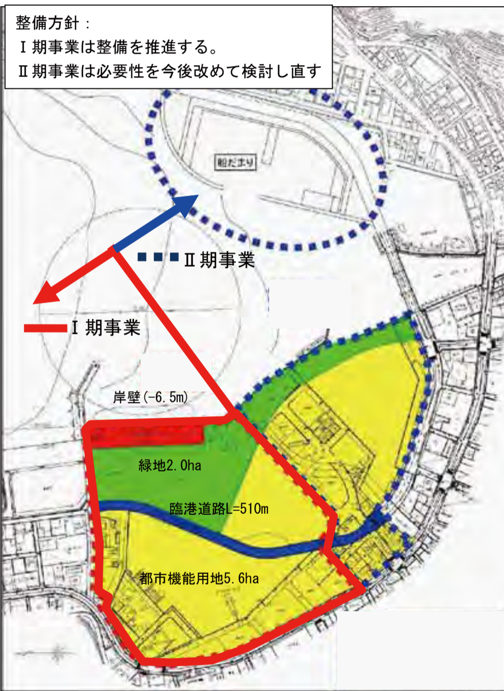
名瀬港本港地区計画平面図
