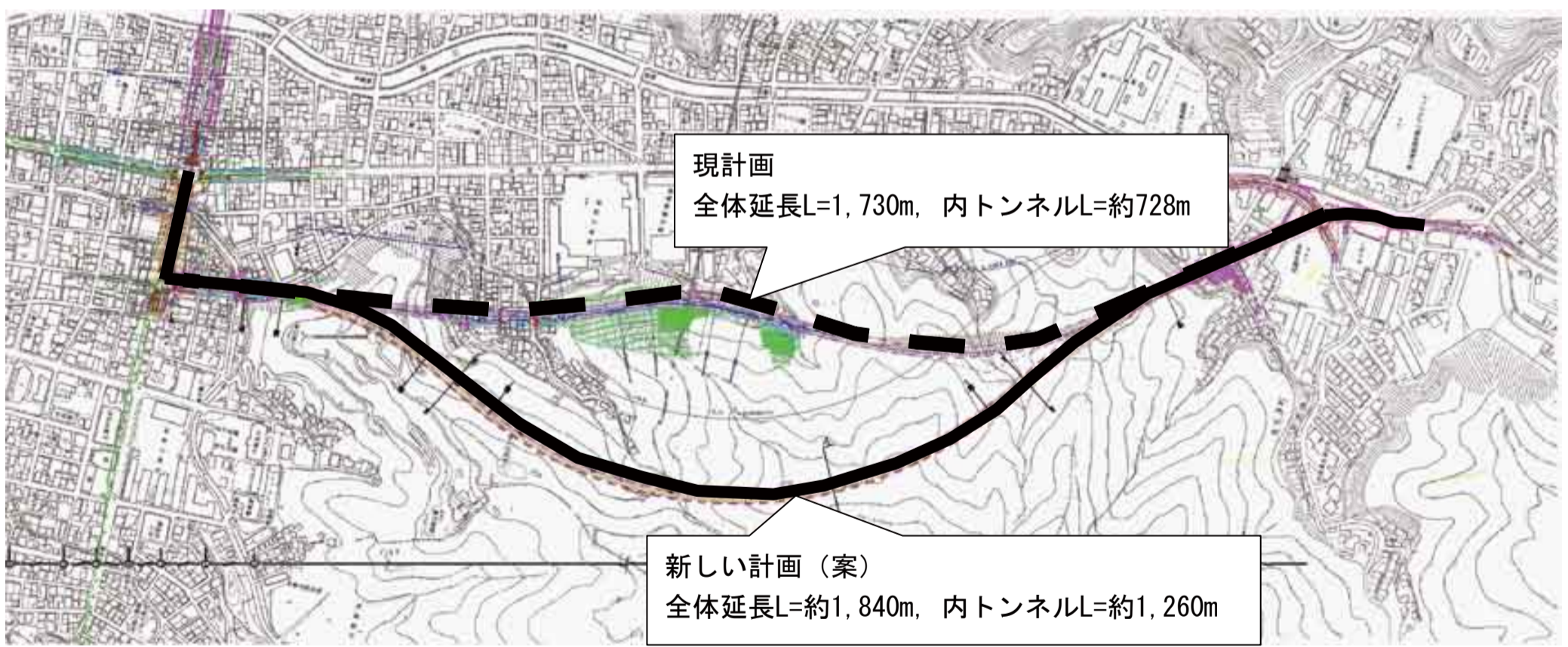
一般国道58号おがみ山バイパス事業現計画(点線)と新しい計画(案)(実線)の比較図
